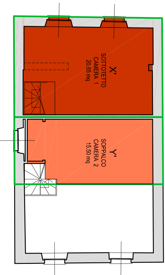
- PIANTA PIANO SOTTOTETTO - scala -
