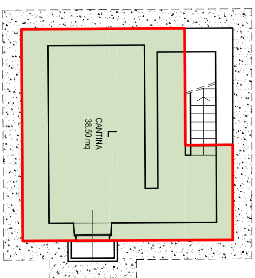
- Pianta Piano Interrato - scala -
